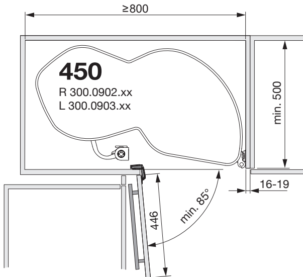
Abbildung: Montage rechts Illustration: Montage à droite Illustration: Right hand mounting
